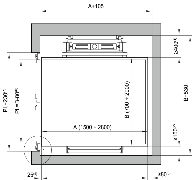
Fosse réduite
