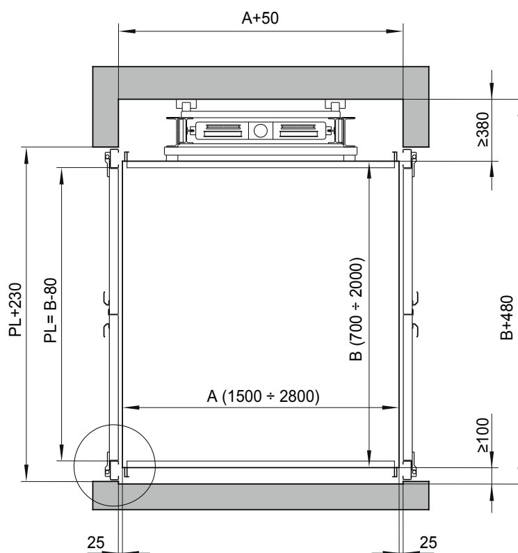
Double accès
