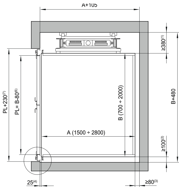
Accès simple lateral
