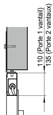
Porte coulissante
