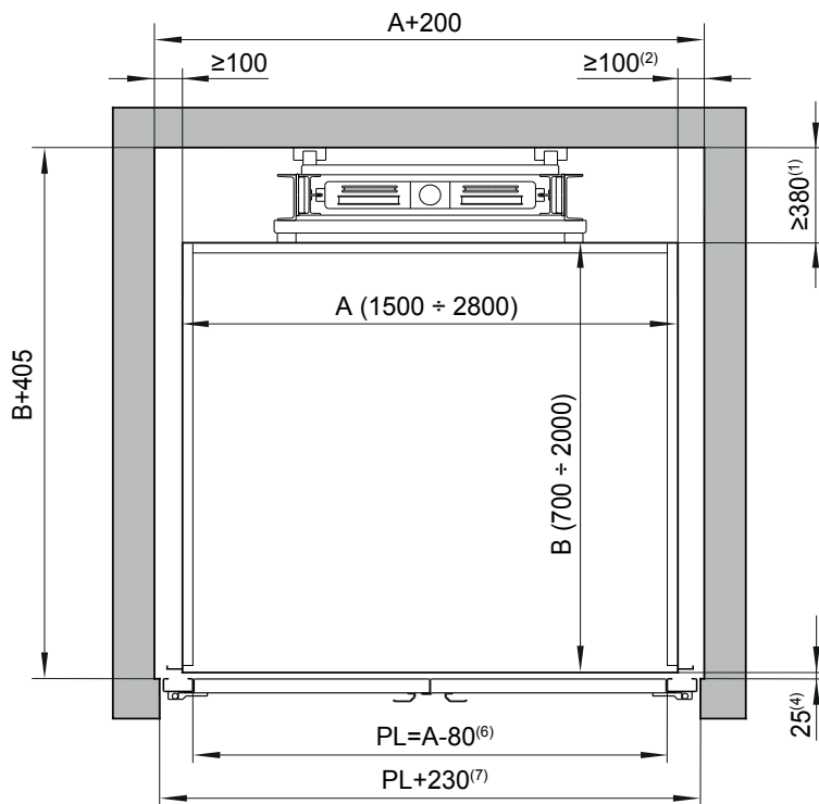
Accès simple frontal
