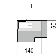
Porte battante
